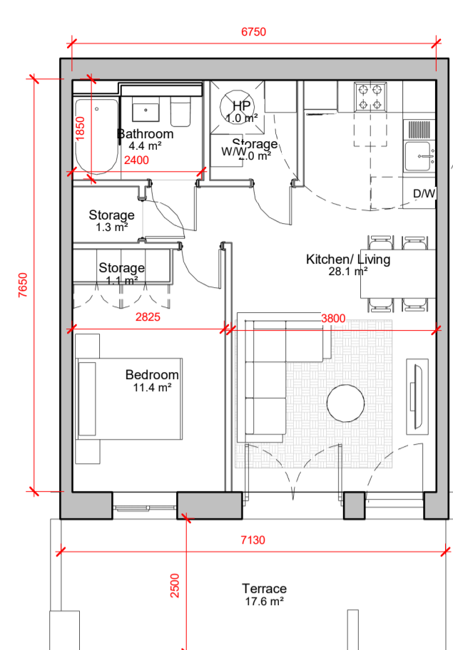
9 1 BED TYPE R 1 : 100
