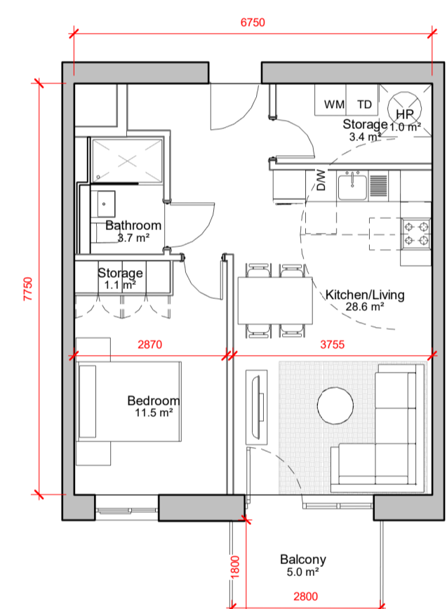
2 1 BED TYPE U 1 : 100
