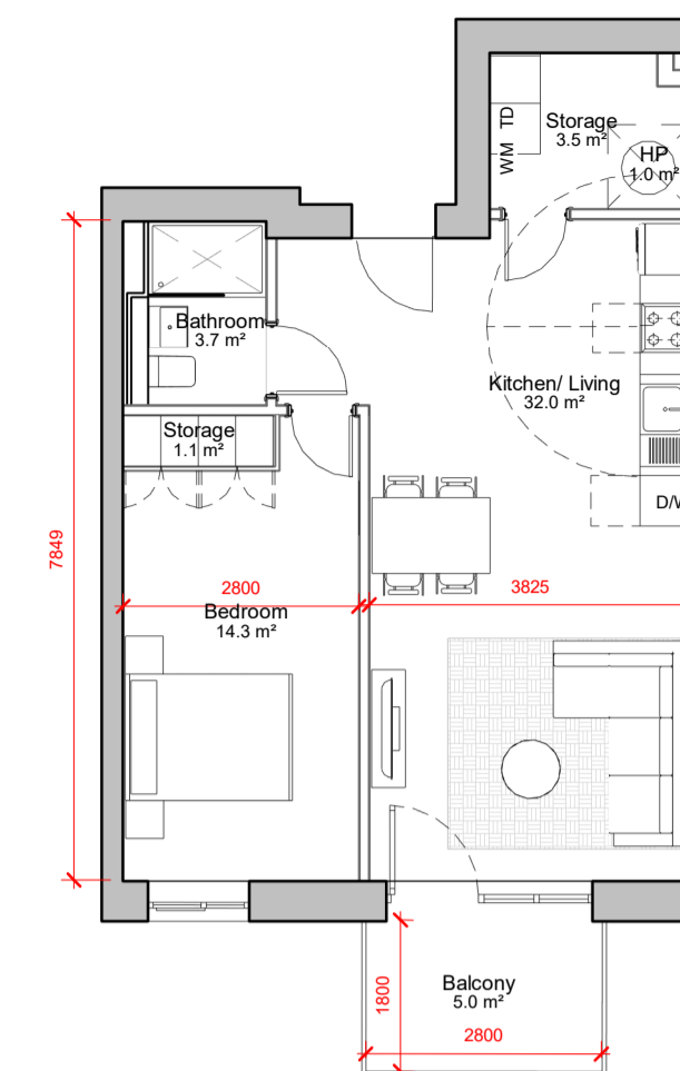
6 1 BED TYPE S 1 : 100
