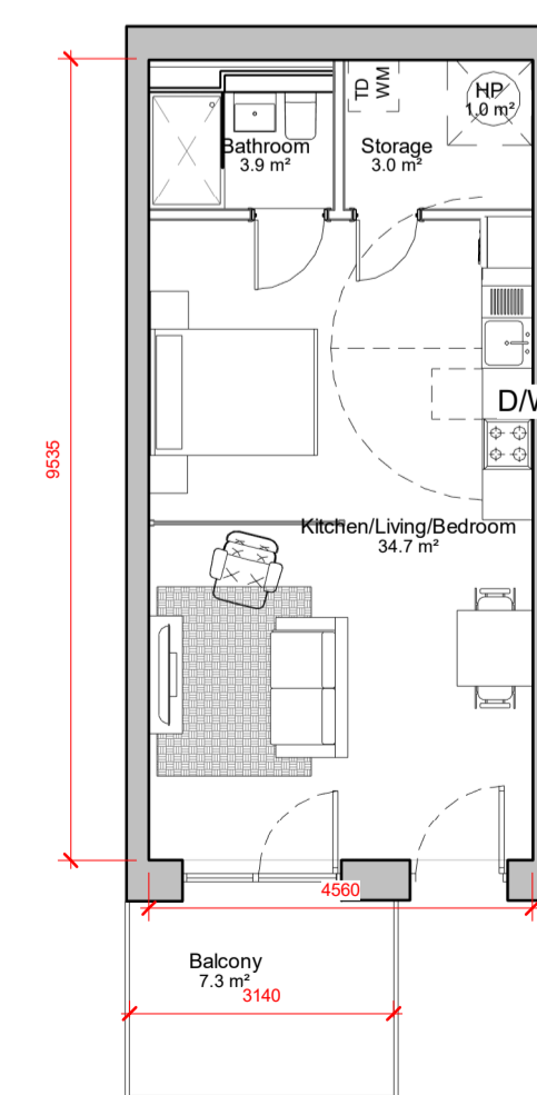
3 1 BED TYPE STUDIO 1 : 100
