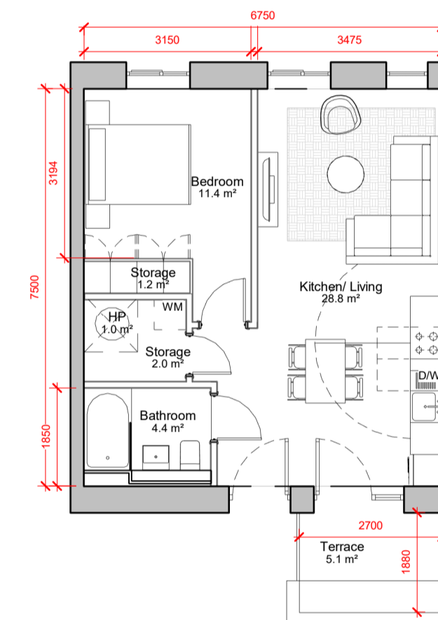
4 1 BED TYPE V 1 : 100
