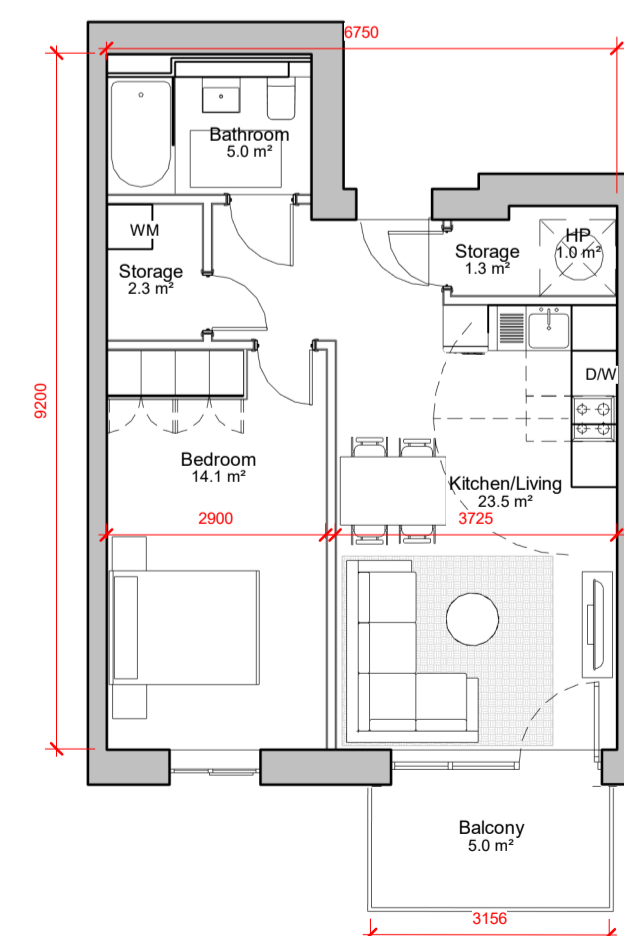
5 1 BED TYPE W1 1 : 100
