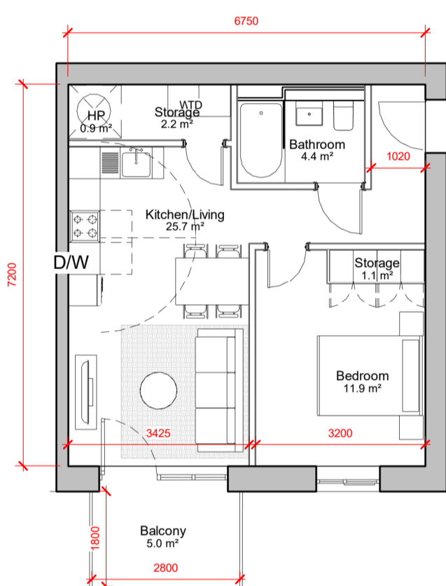
1 1 BED TYPE T 1 : 100
