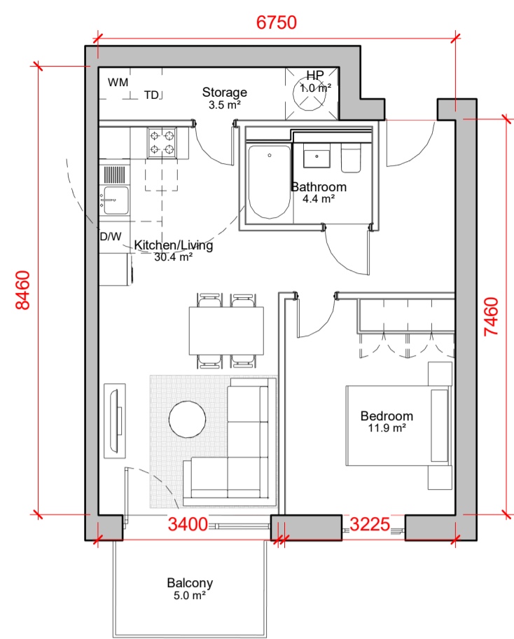
8 1 BED TYPE Q2 1 : 100
